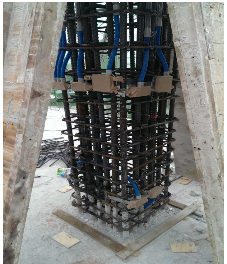
◎ .6F 頂版灌漿、7F 柱. 鋼筋綁紮，柱內配管、牆內配管
