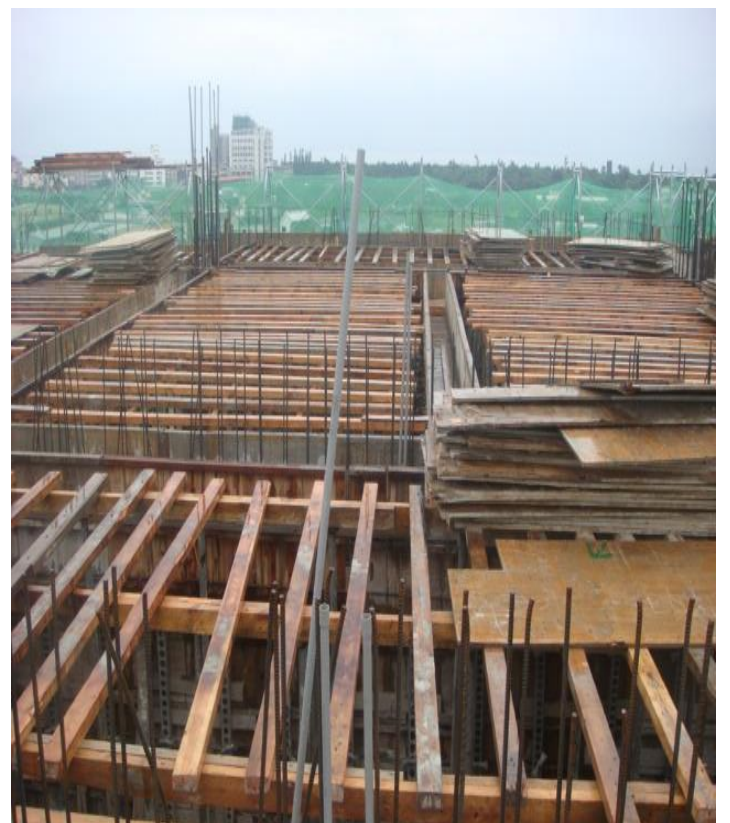
◎ .6F 頂版灌漿、7F 柱. 鋼筋綁紮，柱內配管、牆內配管
